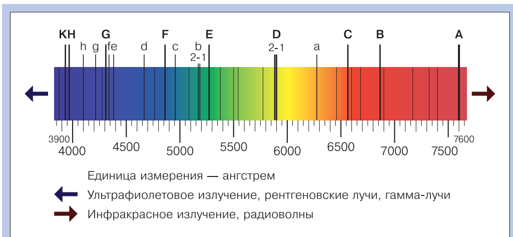
Рис. 135. Положение наиболее сильных тёмных линий в оптическом спектре Солнца от 3900 до 7600 ангстрем. Вверху приведены обозначения линий. Самые заметные линии принадлежат водороду, кальцию, магнию, натрию, железу
