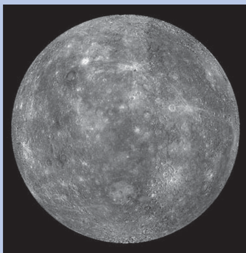
Рис. 88. Фотокарта Меркурия, составленная по снимкам зонда «Мессенджер» (NASA)
