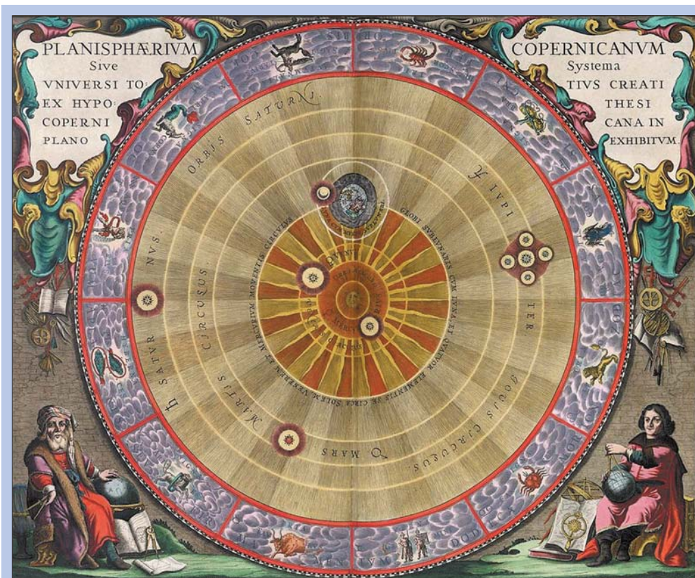
Рис. 65. Гелиоцентрическая система мира
