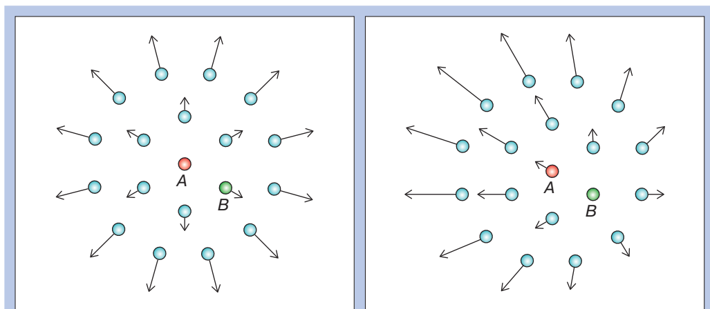
Рис. 189. Скорости галактик для наблюдателей в двух галактиках: A и B . Картина расширения в обоих случаях одинакова
