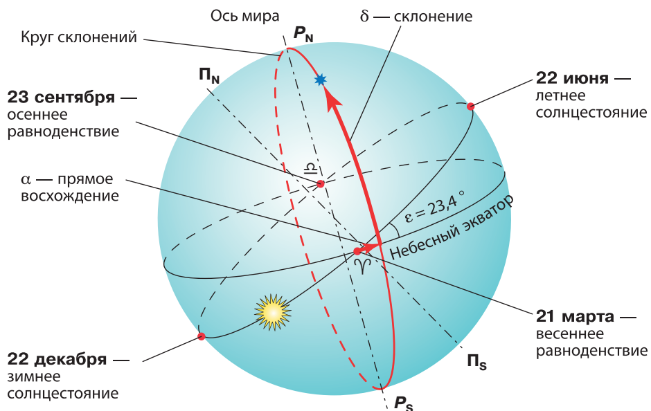
Рис. 49. За начало отсчёта прямого восхождения принята одна из двух точек пересечения небесного экватора с эклиптической — точка весеннего равноденствия ( \gamma ). Линия P_N P_S — это ось эклиптики, параллельная оси земной орбиты
