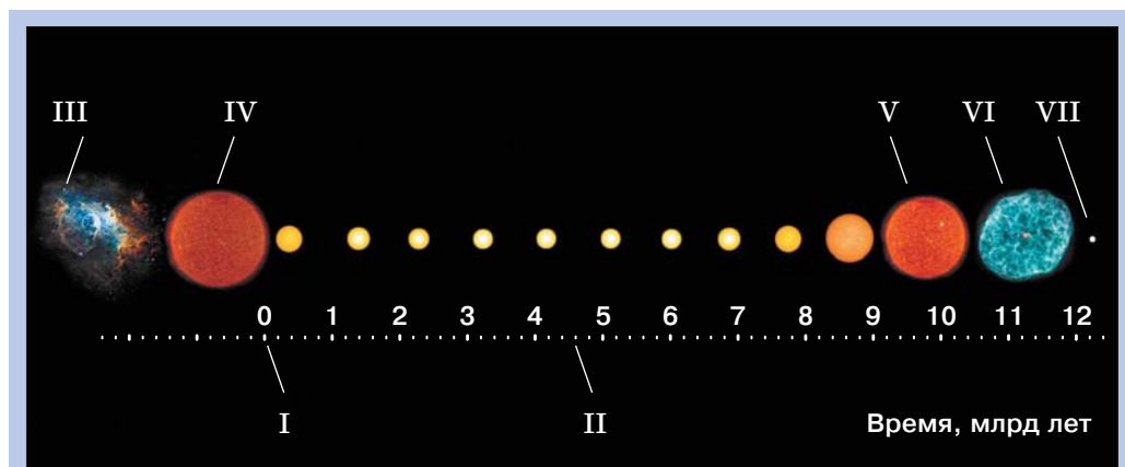
Рис. 150. Эволюция Солнца: I — начало термоядерной реакции; II — настоящее (4,57 млрд лет); III — часть молекулярного облака; IV — протозвезда; V — красный гигант; VI — планетарная туманность; VII — белый карлик
