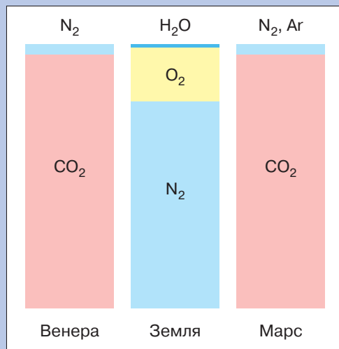
Рис. 90. Состав атмосферы планет земной группы. Меркурий практически лишён атмосферы
