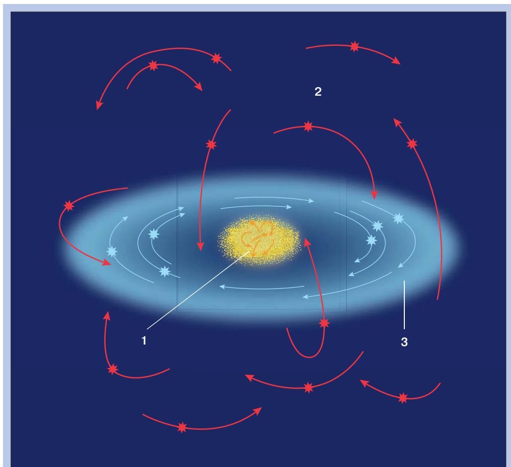
Рис. 162. Движение звёзд в Галактике. Дугами показаны участки орбит звёзд в диске и сферической составляющей: 1 — балдж; 2 — гало; 3 — диск
