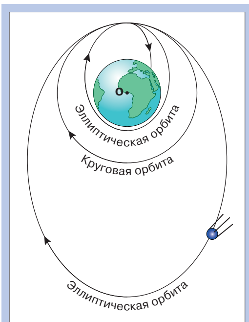
Рис. 72. Орбиты искусственных спутников Земли
