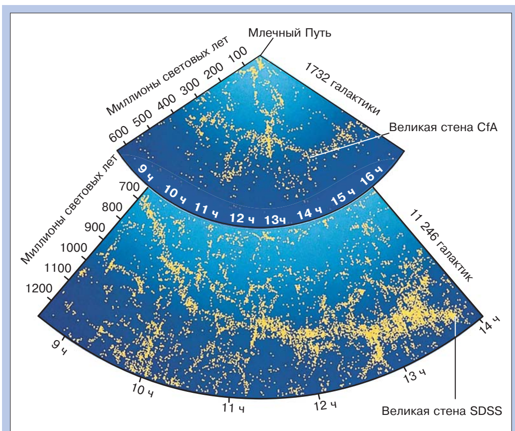
Рис. 193. Крупномасштабное распределение галактик в пространстве в направлении узкого сектора неба по данным обзора SDSS, выполненного в США
