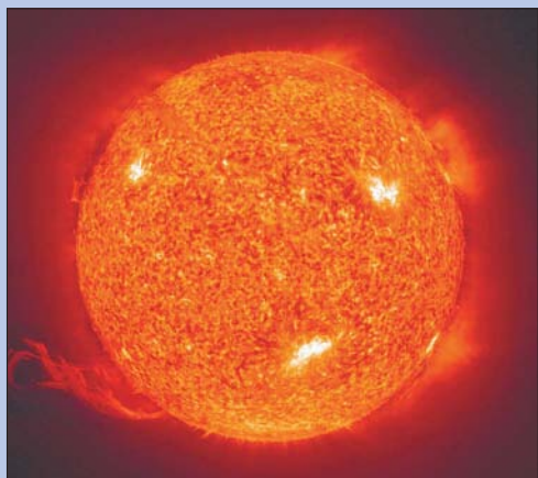
Рис. 142. Гигантский солнечный протуберанец (внизу слева)
