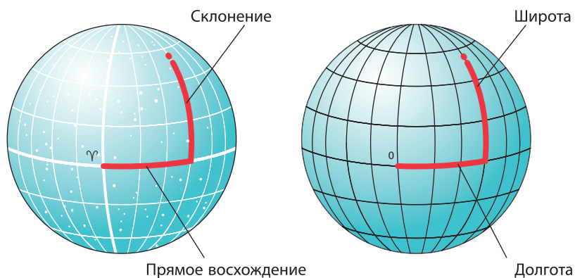
Рис. 50. Небесные экваториальные координаты подобны географическим координатам на Земле
