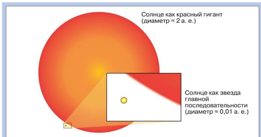
Рис. 151. Солнце на стадии красного гиганта многократно увеличит размер своей фотосферы и, возможно, достигнет орбиты Земли
