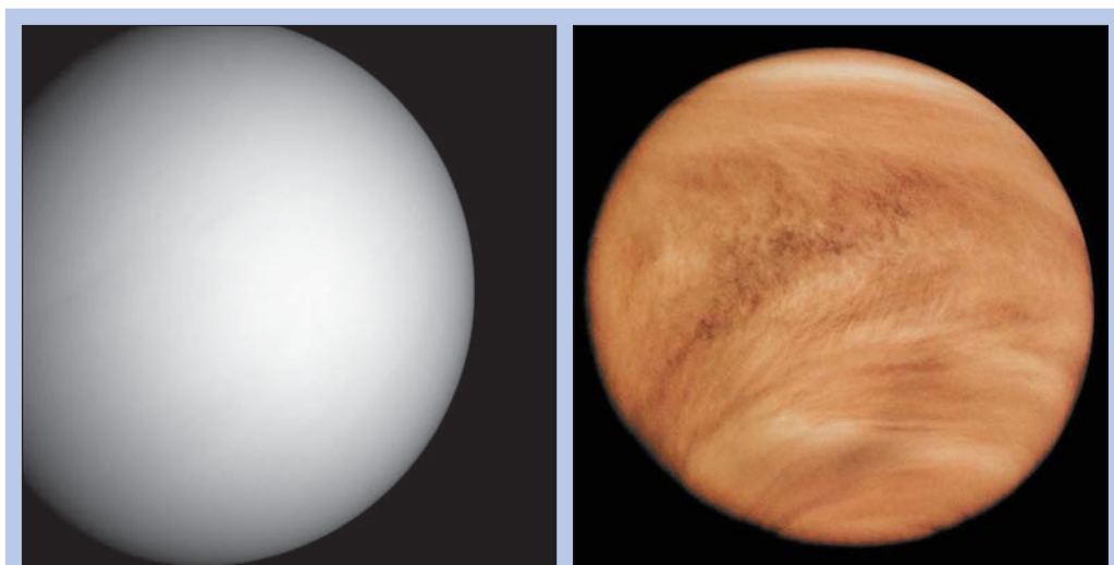
Рис. 92. Слева: Венера в диапазоне видимого света. Так воспринимает её человеческое зрение. Фото зонда «Маринер-10» (NASA). Справа: Венера в ультрафиолетовом диапазоне, более чётко выделяющем структуру облаков. Фото зонда «Пионер-Венера» (NASA)
