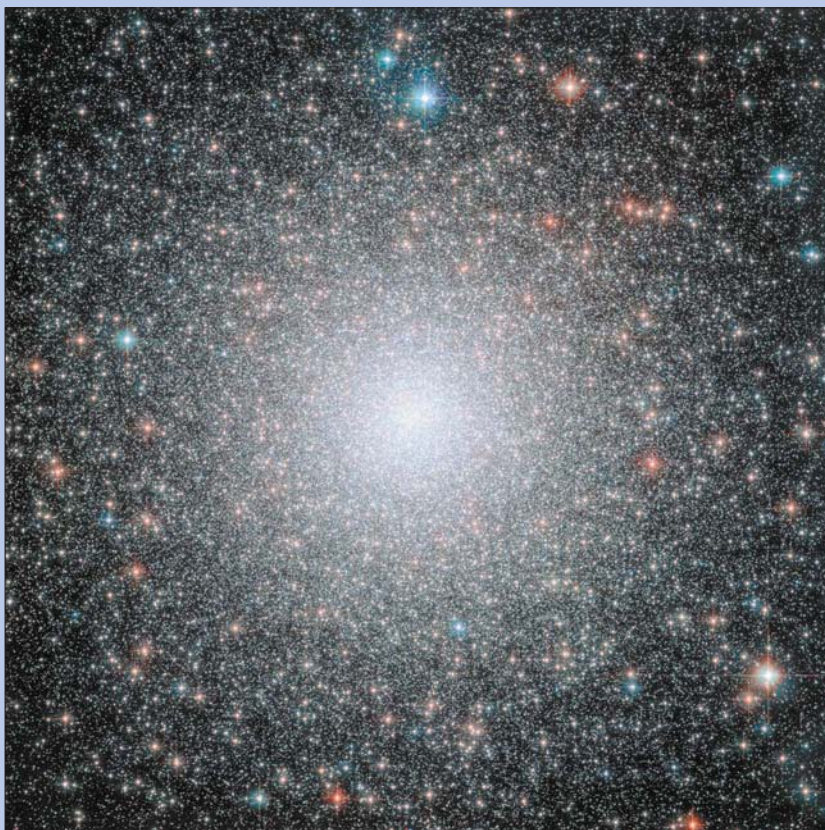
Рис. 161. Шаровое звёздное скопление NGC 6388
