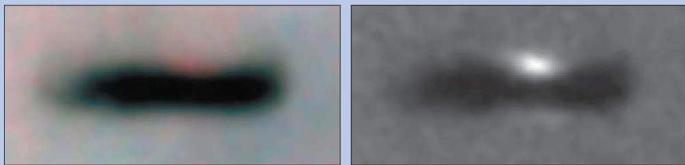
Рис. 175. Формирующиеся звёзды, окружённые непрозрачными газовой-пылевыми (протопланетными) дисками, в области Туманности Ориона
