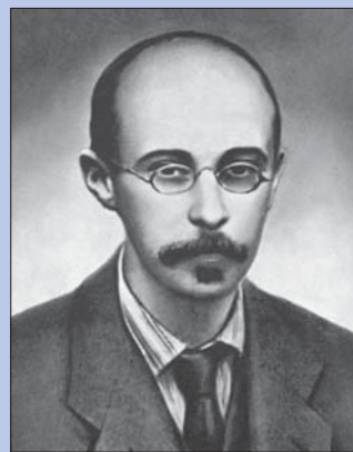
Рис. 190. Александр Александрович Фридман (1888—1925)
