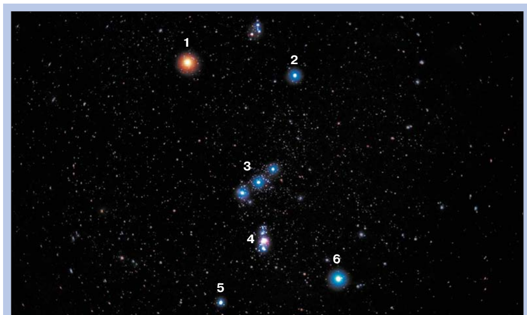
Рис. 166. Положение Туманности Ориона в созвездии Орион: 1 — Бетельгейзе; 2 — Беллатрикс; 3 — Пояс Ориона; 4 — Туманность Ориона; 5 — Саиф; 6 — Ригель
