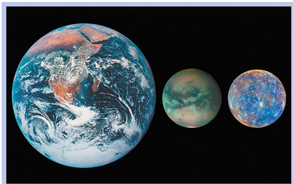
Рис. 99. Сравнительные размеры Земли, Титана и Меркурия. Все три изображения реальные, цветовой контраст усилен
