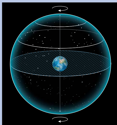
Рис. 36. Видимое вращение небесной сферы для наблюдателя на Северном полюсе
