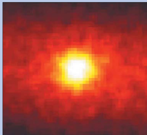
Рис. 148. Изображение Солнца в нейтринных «лучах»
