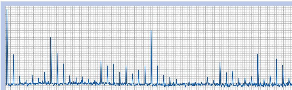
Рис. 154. Запись радиоимпульсов первого пульсара PSR 1919+21 с периодом 1,3373 с на частоте 72,7 МГц
