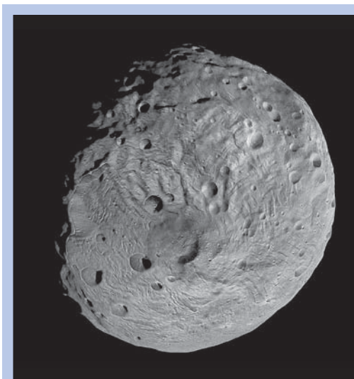
Рис. 106. Астероид Веста. Вид со стороны южного полюса. Фото зонда «Рассвет» (Dawn, NASA)
