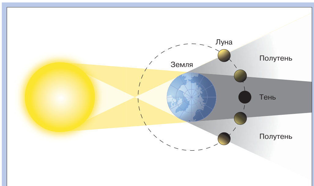
Рис. 61. Схема лунного затмения
