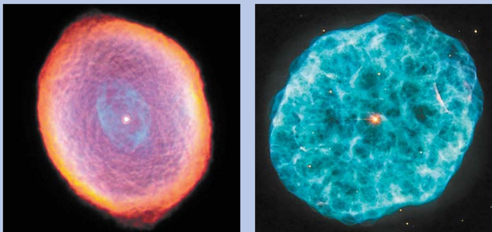
Рис. 152. Слева: планетарная туманность IC 418. Справа: планетарная туманность NGC 1501. IC — Index Catalogue, NGC — New General Catalogue
