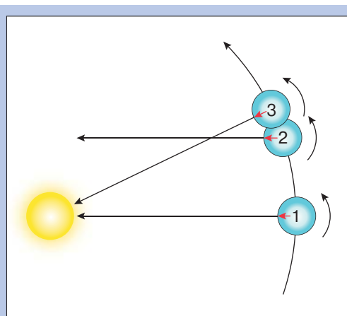
Рис. 53. Объяснение различия звёздных и солнечных суток
