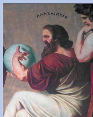
Рис. 3. Анаксагор (ок. 500 до н. э. — 428 до н. э.)
