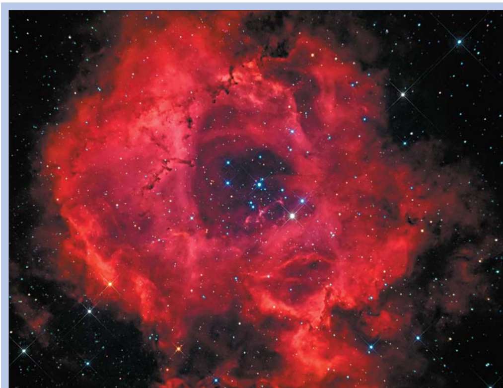
Рис. 173. Эмиссионная туманность Розетка (NGC 2237). Свечение газа вызвано его нагревом горячими звёздами, недавно сформировавшимися в центре облака
