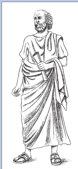
Рис. 5. Аристарх Самосский (III в. до н. э.)
