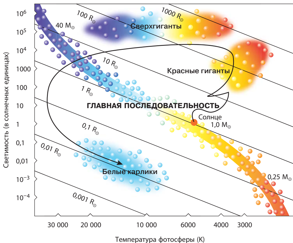
Рис. 153. Эволюционный трек звезды массой 1 M_{\odot}
