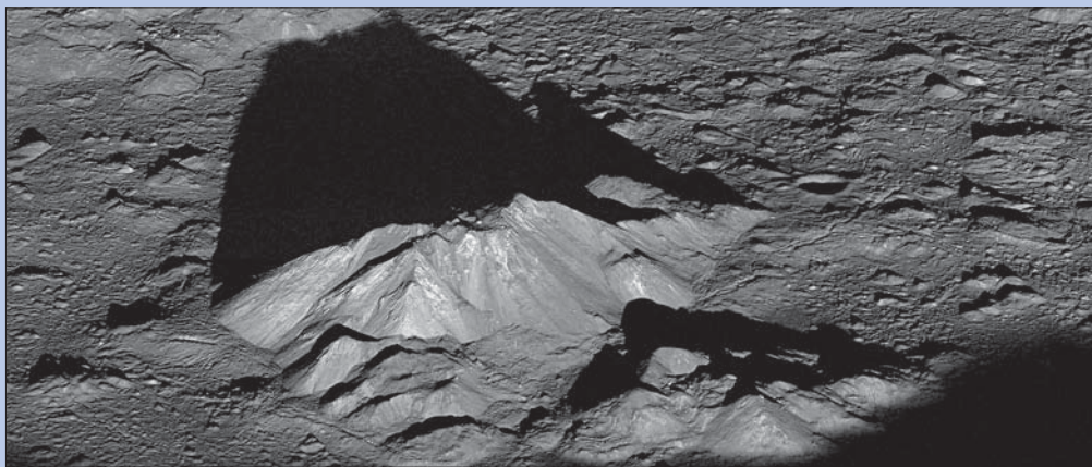
Рис. 85. Центральный пик в кратере Тихо. Дно кратера лежит на глубине 4,8 км, а центральная гора возвышается на 2 км над уровнем дна. Протяжённость снимка слева направо около 15 км. Фото LRO (NASA)
