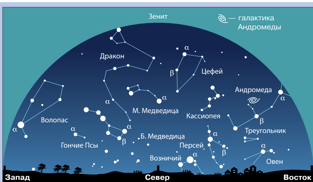
Рис. 32. Полярные созвездия сентябрьским вечером
