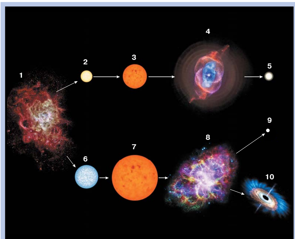
Рис. 156. Эволюция звёзд разной массы: 1 — газОВО-пылевое облако; 2 — звезда солнечной массы; 3 — красный гигант; 4 — планетарная туманность; 5 — белый карлик; 6 — массивная звезда; 7 — красный сверхгигант; 8 — взрыв сверхновой; 9 — нейтронная звезда; 10 — чёрная дыра, окружённая аккреционным диском
