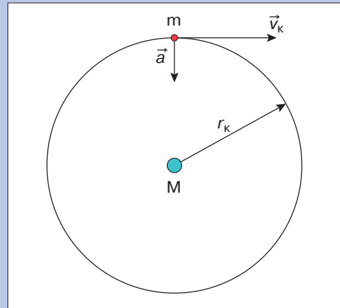
Рис. 71. Схема кругового движения тела
