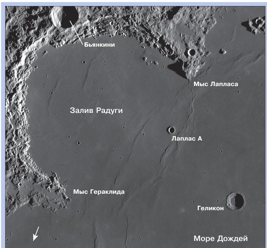
Рис. 83. Залив Радуги на Луне. Сторона кадра 360 км. Стрелкой показано положение «Лунохода-1»
