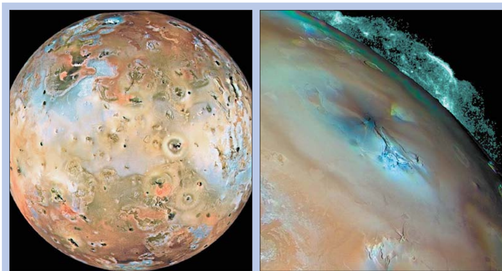
Рис. 97. Слева: спутник Юпитера Ио. Справа: извержение одного из вулканов на Ио, скрытого за горизонтом. Фото зонда «Галилео» (NASA)
