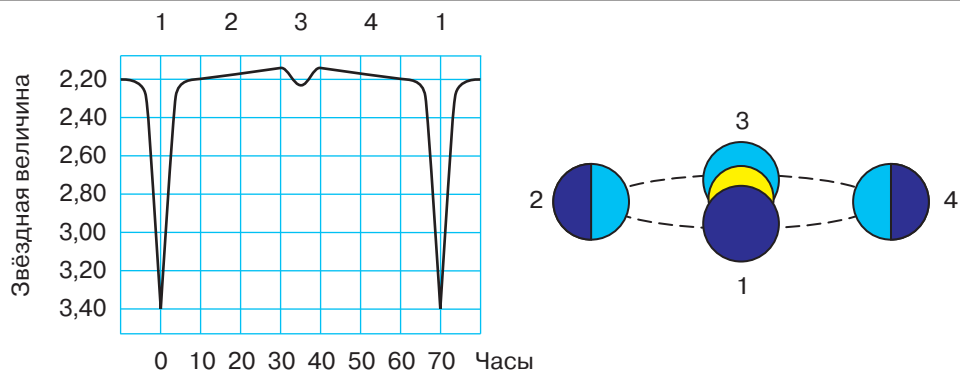
Рис. 157. График изменения яркости Алголя и четыре взаимных положения его компонентов в характерные моменты орбитального цикла
