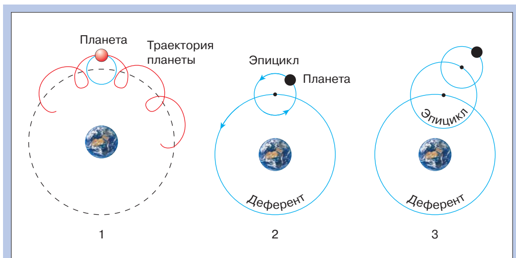
Рис. 63. Система эпициклов по Птолемею: 1 — понятное движение планеты позволяет смоделировать один эпицикл; 2 — простая модель с одним эпициклом; 3 — более сложная модель с двумя эпициклами
