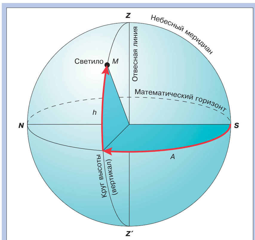
Рис. 47. Горизонтальная система координат
