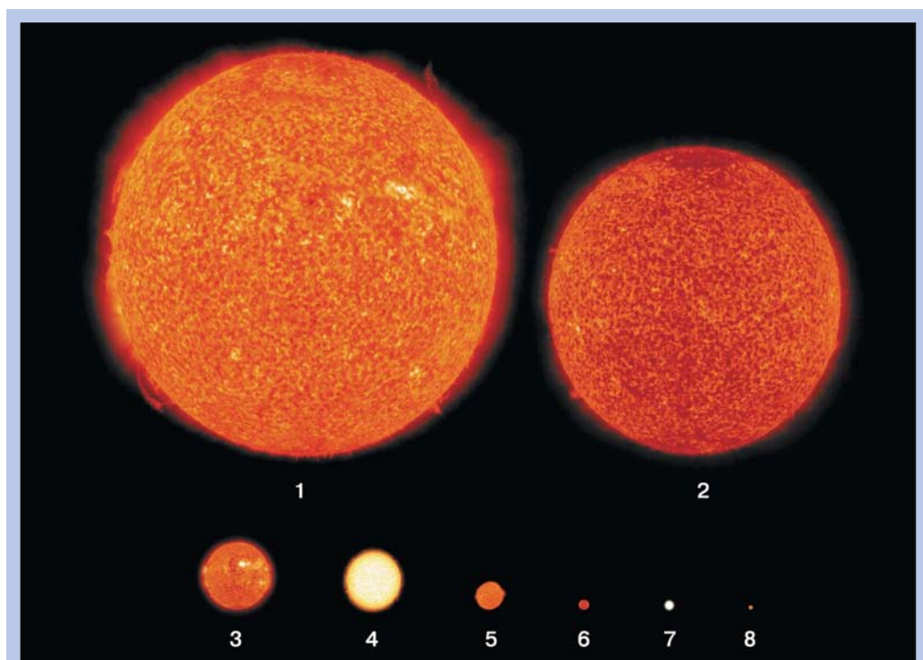
Рис. 145. Сравнительные размеры звёзд-гигантов и Солнца: 1 — Бетельгейзе; 2 — Антарес; 3 — Альдебаран; 4 — Ригель; 5 — Арктур; 6 — Поллукс; 7 — Сириус; 8 — Солнце
