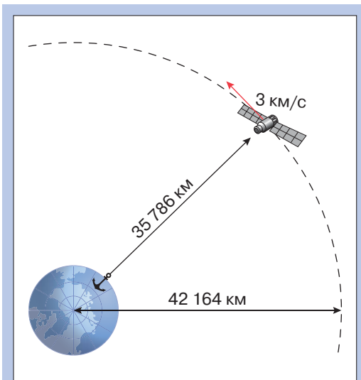
Рис. 75. Геостационарная орбита
